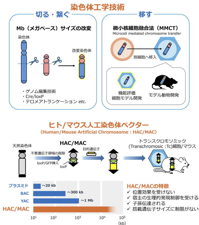
（上）染色体工学技術の概要（下）ヒト/マウス染色体ベクターとその特徴
